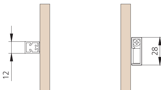
Öntapadós díszosztó profil
