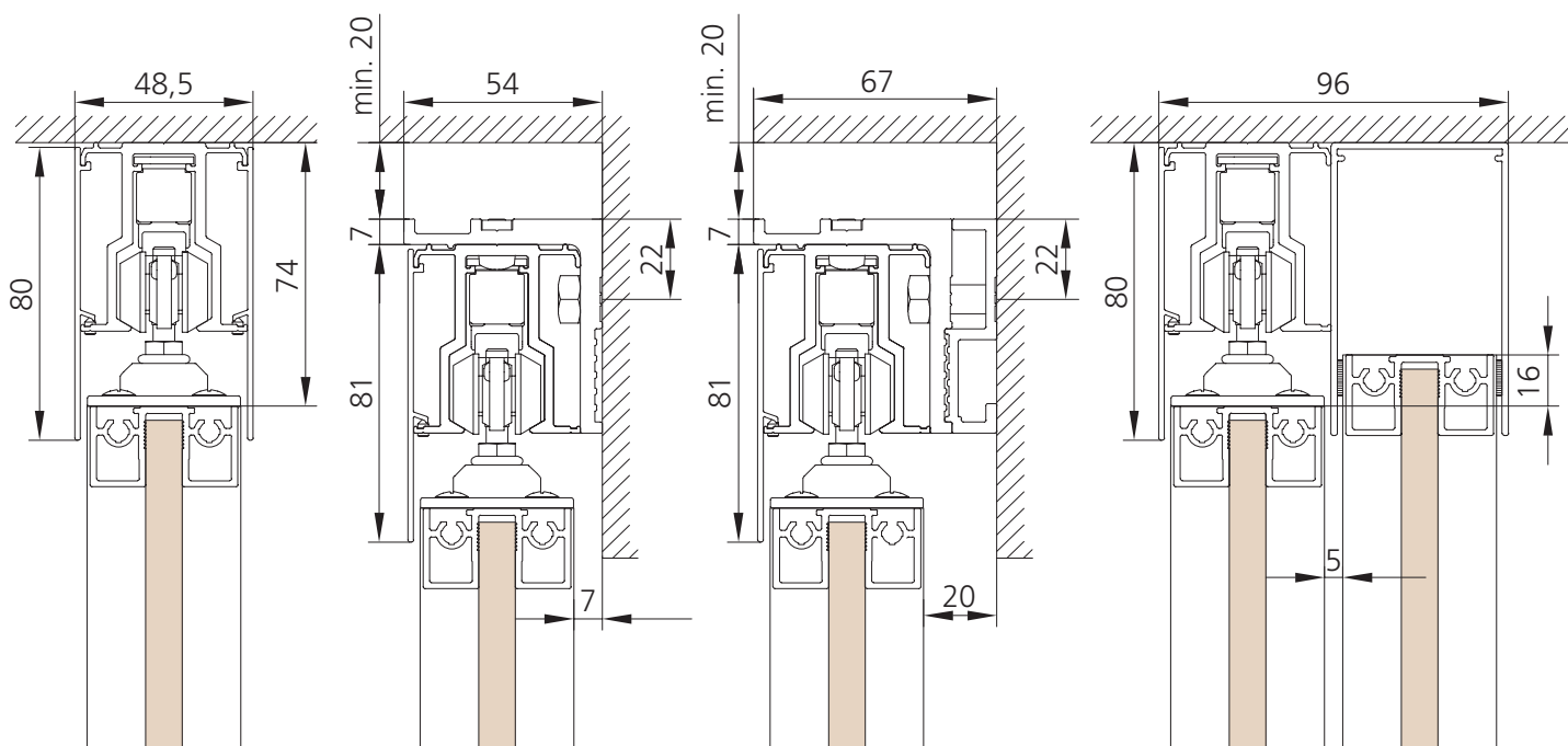
Felső sín rögzítési lehetőségek
